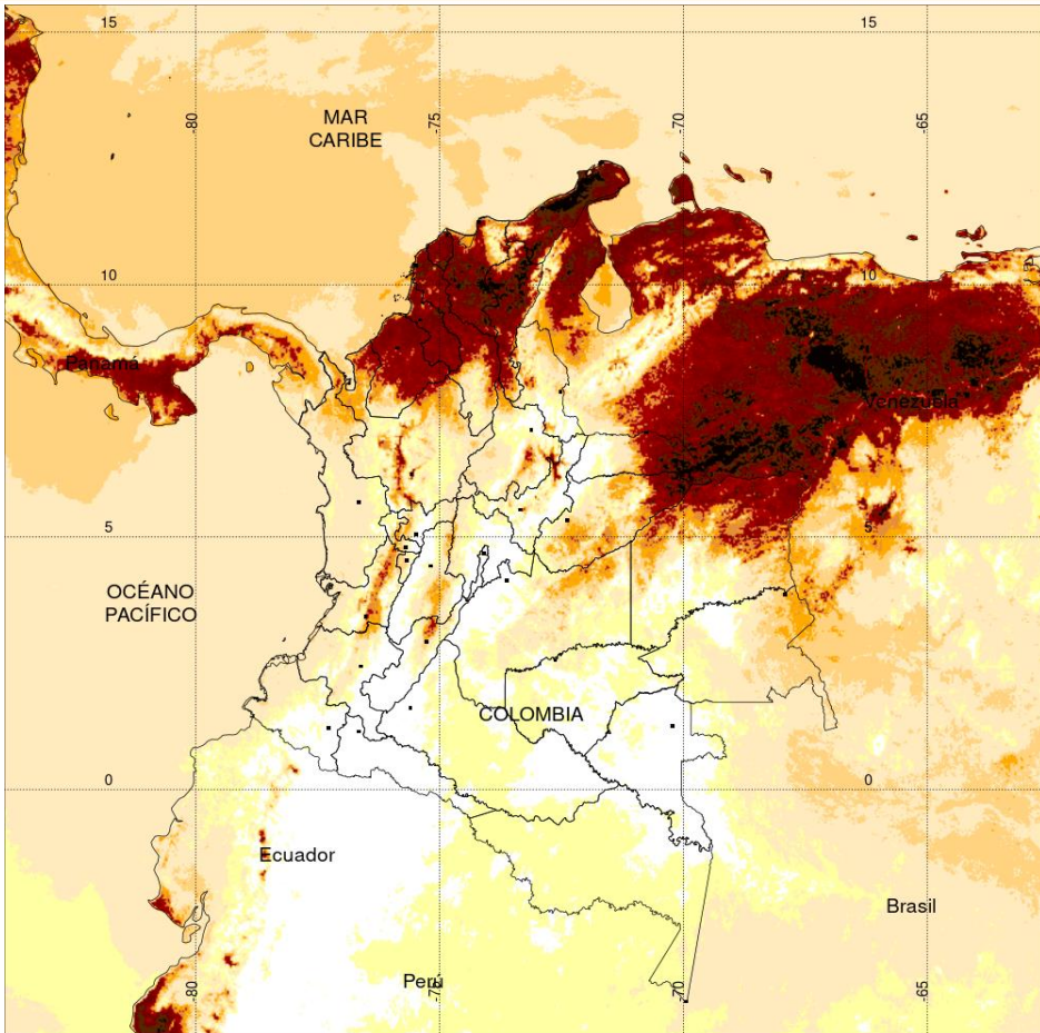
TEMPERATURA SUPERFICIAL MÁXIMA POR ESTIMACIÓN SATELITAL (GOES-16) ( 2020-04-17 09:00:00 a 2020-04-17 18:30:00 )
