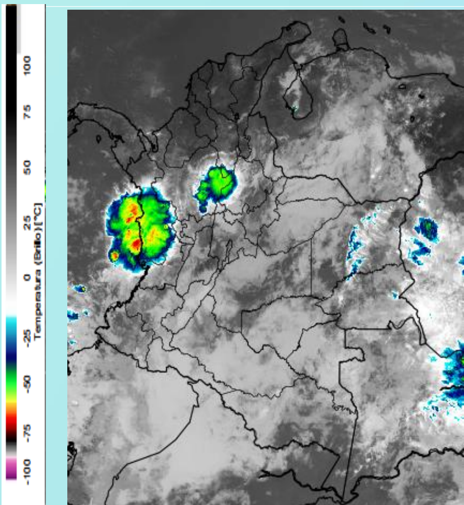
Imagen GOES East Canal Infrarrojo, 18 de abril de 2020. Hora 08:20 HLC. Fuente: IDEAM-GOES 16
