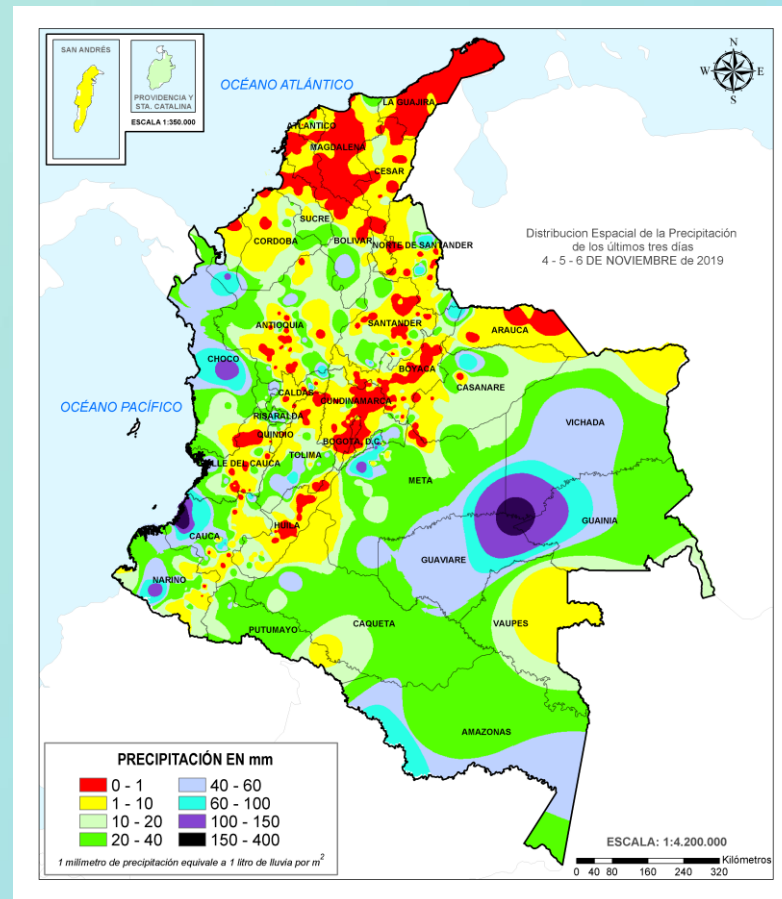
Precipitación últimas 72 horas desde las 7:00 HLC del lunes 4 y hasta las 7:00 HLC del jueves, 7 de noviembre de 2019 Fuente: IDEAM
