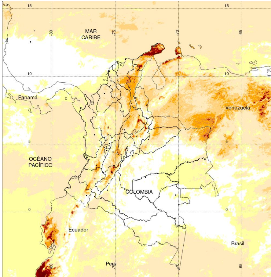
TEMPERATURA SUPERFICIAL MÁXIMA POR ESTIMACIÓN SATELITAL (GOES-16) (2019-11-06 09:00:00 a 2019-11-06 18:30:00)
