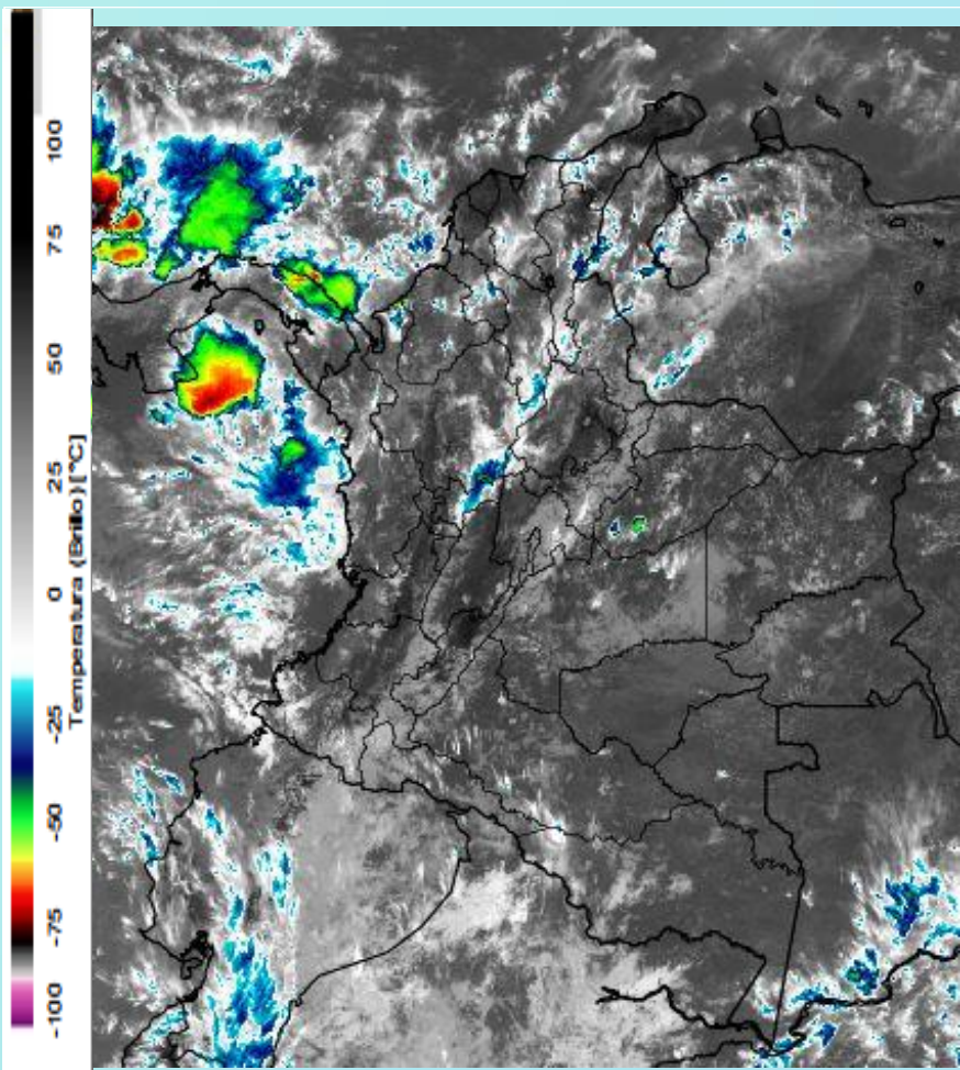
Imagen GOES East Canal Infrarrojo 7 de noviembre de 2019. Hora 11:20 HLC. Fuente: IDEAM-GOES 16
