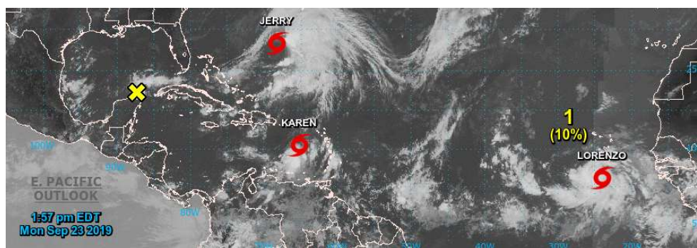
Figura 1. Ubicación de la tormenta tropical KAREN en el mar Caribe. Fuente: National Hurricane Center (NHC).
