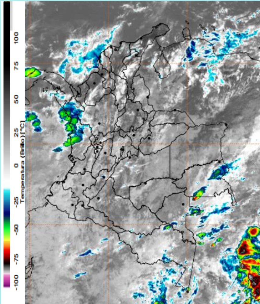
Imagen GOES East Canal Infrarrojo, 17 de diciembre de 2021. Hora 11:20 HLC. Fuente: IDEAM-GOES 16
