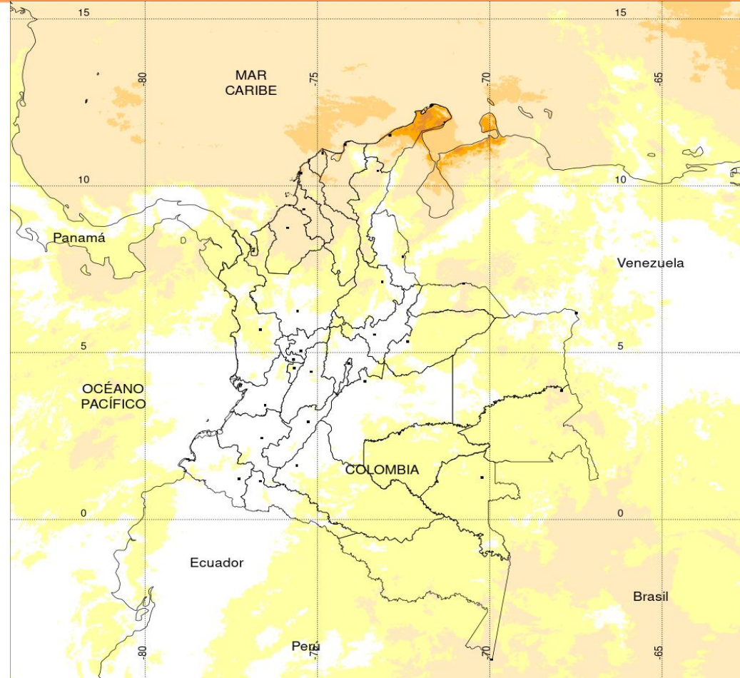
TEMPERATURA SUPERFICIAL MÁXIMA POR ESTIMACIÓN SATELITAL (GOES-16) ( 2021-08-09 02:20:00 a 2021-08-09 07:50:00 )
