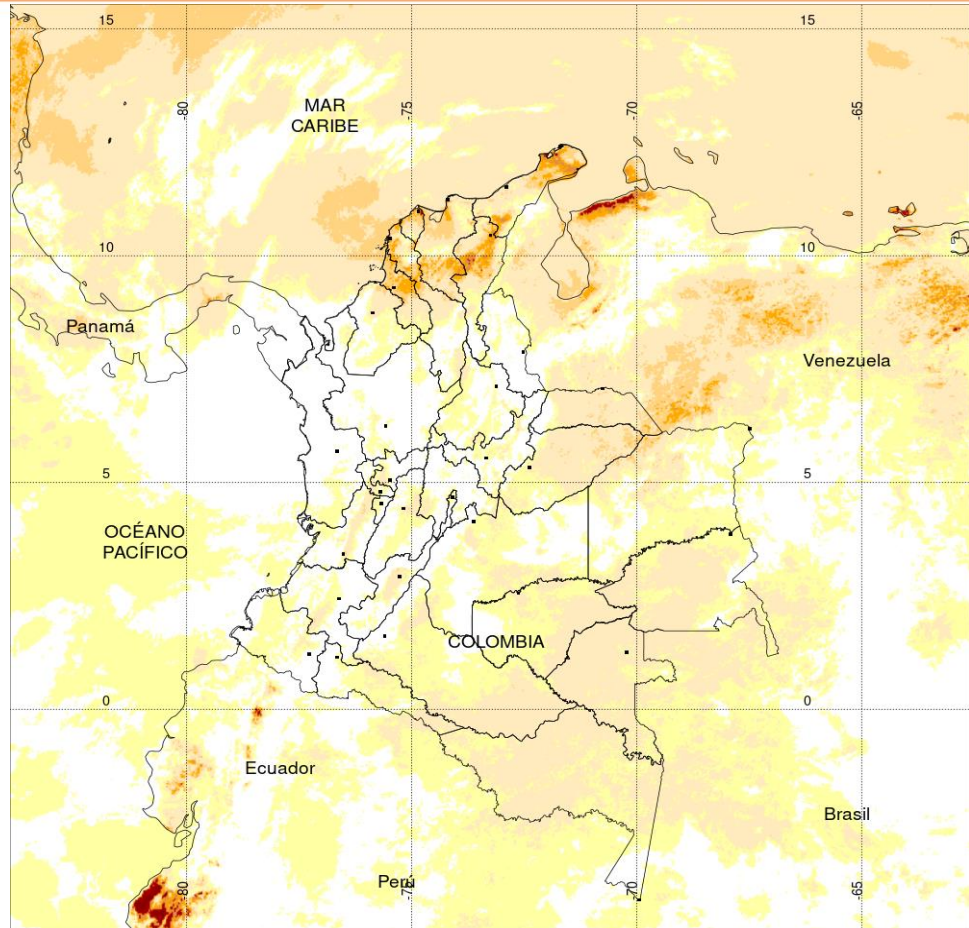
TEMPERATURA SUPERFICIAL MÁXIMA POR ESTIMACIÓN SATELITAL (GOES-16) ( 2020-12-07 09:00:00 a 2020-12-07 11:10:00 )
