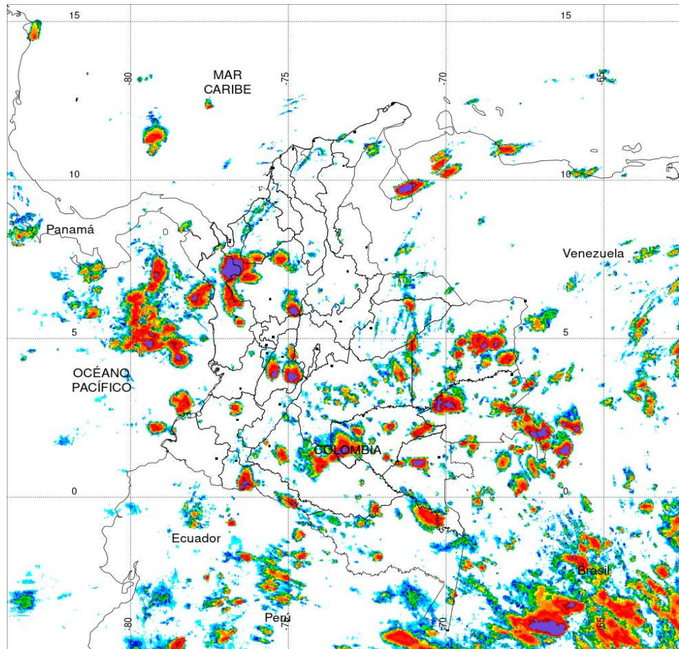
PRECIPITACIÓN TOTAL ACUMULADA POR ESTIMACIÓN SATELITAL (GOES-16) DEC 06 DE 2020 (7:00) - DEC 07 DE 2020 (7:00)
