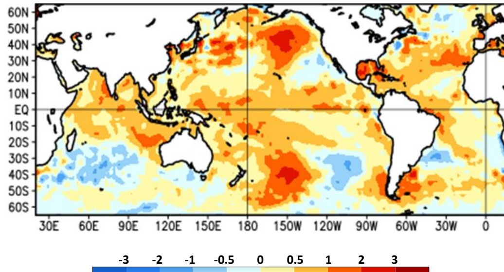
Figura 3. Promedio de las Anomalías de la Temperatura Superficial del Mar (°C), entre el 05 de abril y el 02 de mayo de 2020. Fuente: NOAA
