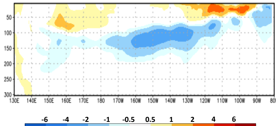
Figura 4. Anomalías de la Temperatura Subsuperficial del Mar (°C), pentada centrada el 28 de abril de 2020. Fuente: NOAA
