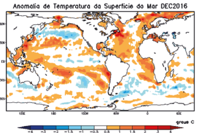
Gráfico 1. Anomalia de la TSM en el océano Pacífico Tropical, para el mes de diciembre de 2016. En gran parte de la cuenca se observan condiciones muy cercanas al ENSO – Neutral. Los colores azules señalan anomalías negativas (enfriamiento), siendo leve en la gama clara y fuerte en tonalidades oscuras, mientras que los blancos definen condiciones de neutralidad y los colores naranjas condiciones de calentamiento. Fuente: Centro de Previsão de Tempo e Estudos Climáticos – CPTEC-INPE (enlace web: http://enos.cptec.inpe.br/ ).
